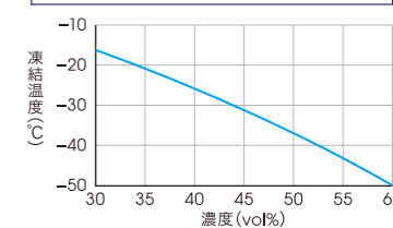
ロングライフクーラントの濃度と凍結温度の関係
